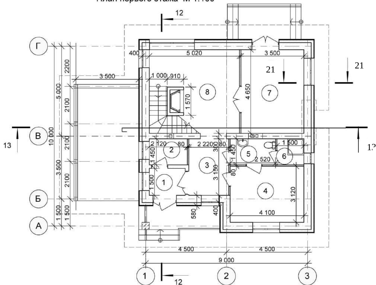
Экспликация помещений
