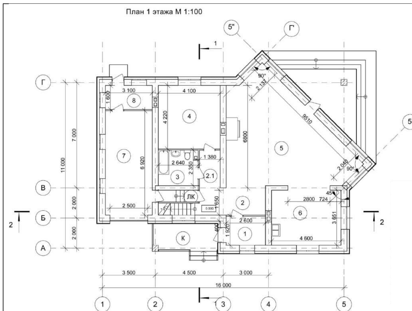
Экспликация 1 этажа
