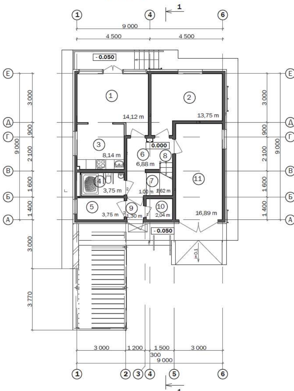
Экспликация помещений на отм. 0,000
